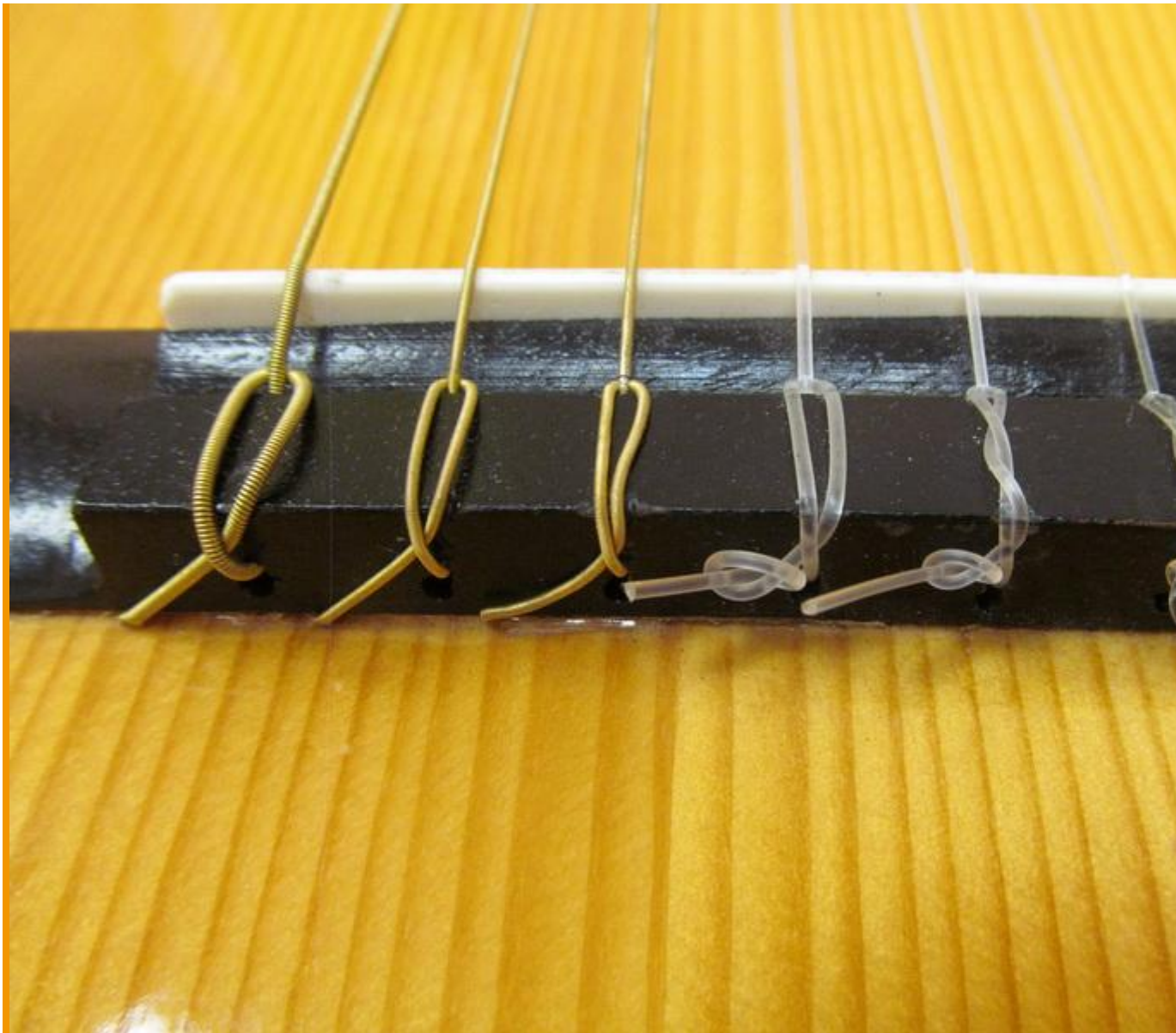
Крепление струн снизу на классике(Рис. 3)
